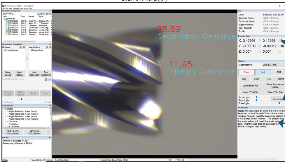
290倍放大倍率下的主副后角
